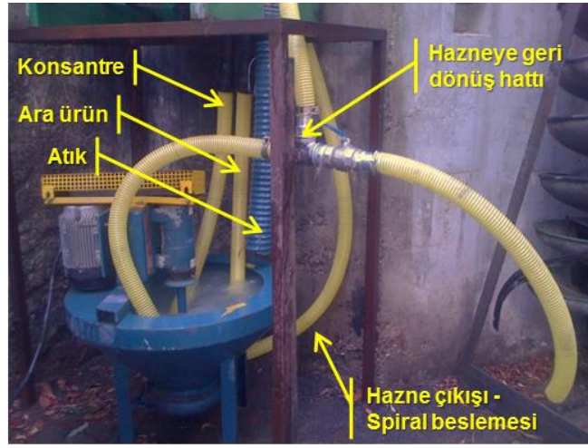
Şekil 6.3: Spiral haznesi ve ürün çıkışları
