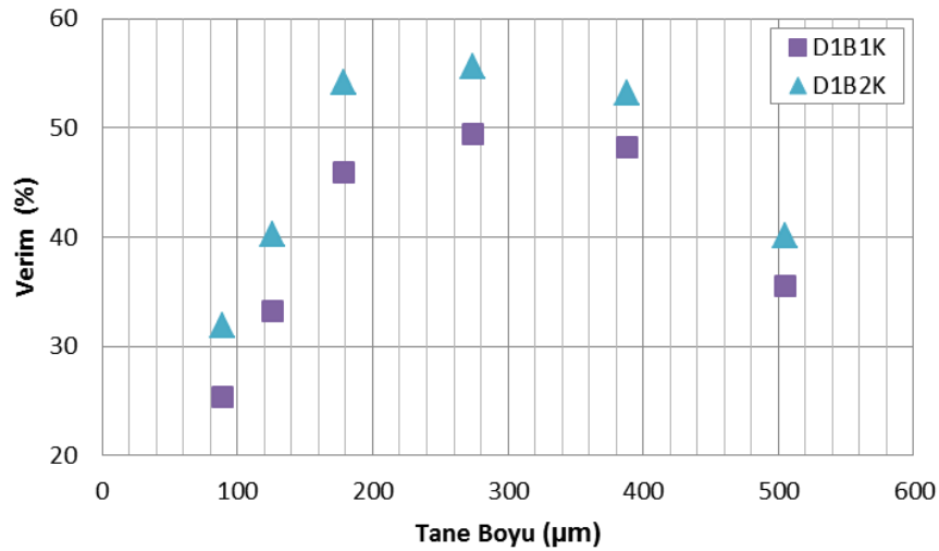
řekil 7.1: Kromit beslemesinin debi 1 kořulunda alınan konsantrelerine ait tane boyu bazında verim sonuları
